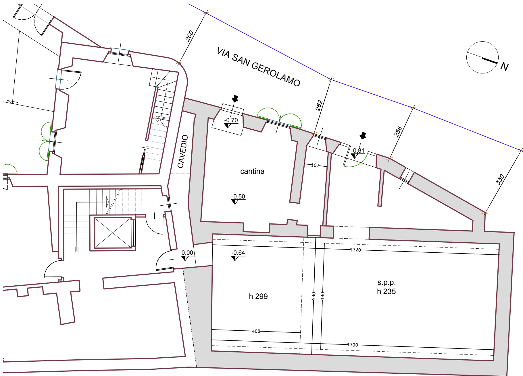
PIANTA PIANO SOTTOSTRADA STATO DI FATTO
