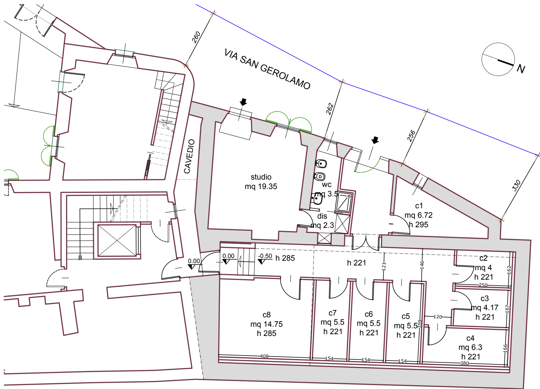
PIANTA PIANO SOTTOSTRADA PROGETTO
